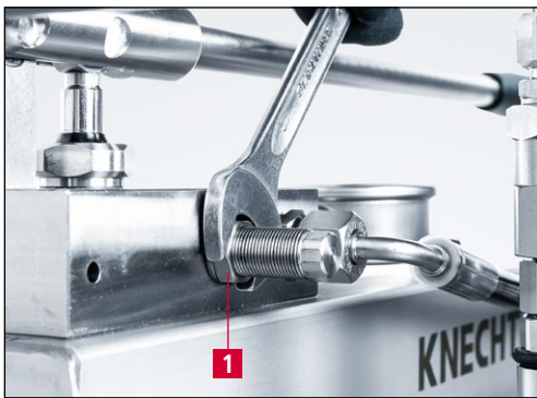
Bild 5-28 Kontermutter festziehen
