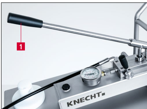
Bild 5-5 Hydraulikdruck aufbauen
