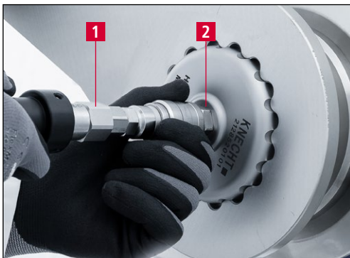
Bild 5-10 Schnellkupplung aufsetzen
