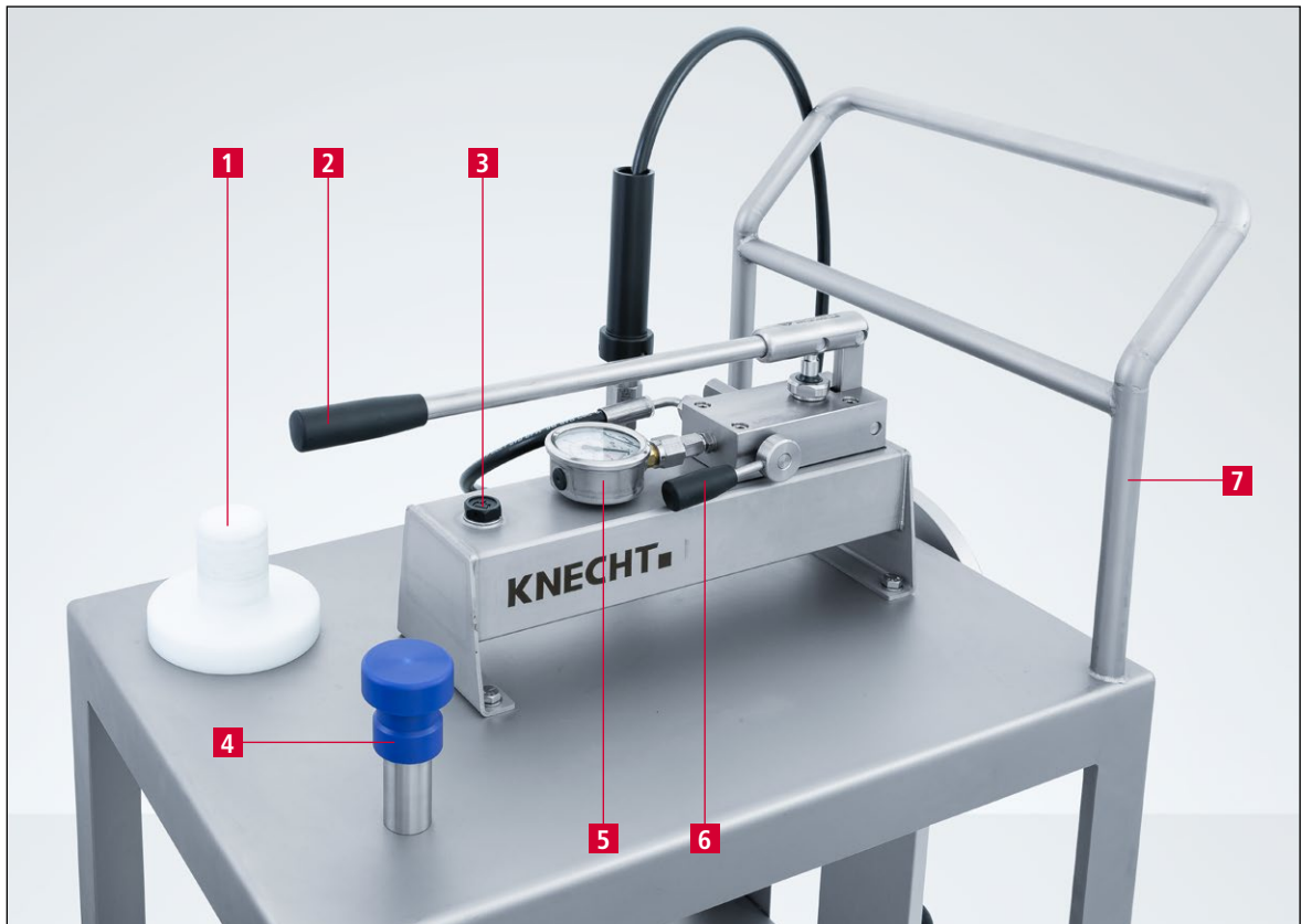
Bild 3-2 Hydraulikwagen mit Hydraulikpumpe
