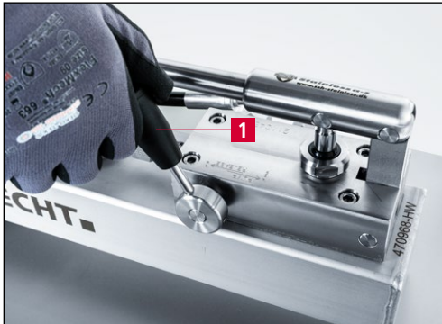
Bild 5-4 Pumpenventil schließen
