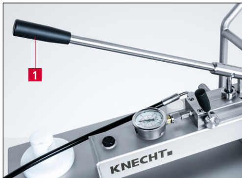
Bild 5-12 Hydraulikdruck aufbauen
