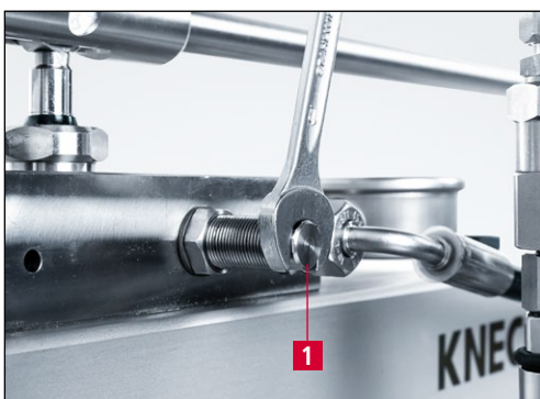
Bild 5-23 Regulierschraube einstellen
