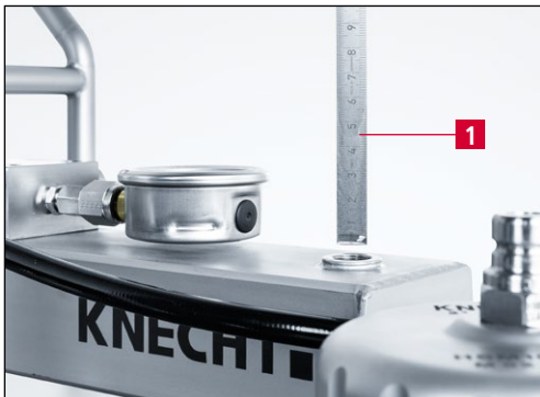
Bild 5-20 Ölstand prüfen
