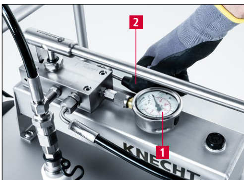
Bild 5-26 Druckwert ablesen
