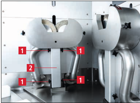
Bild 7-20 Polierpaste wechseln
