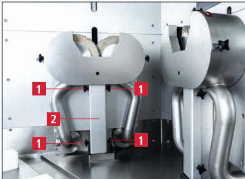
Bild 7-20 Polierpaste wechseln
