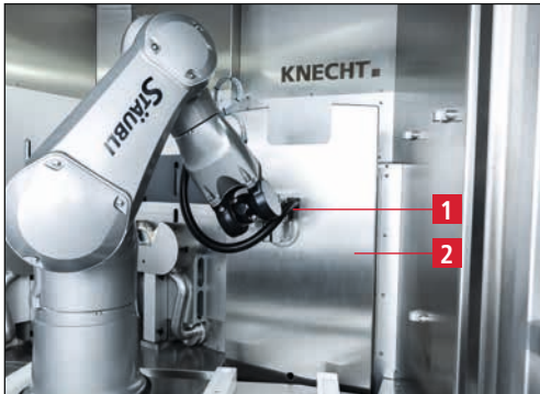
Bild 7-6 Nass-Schleifband wechseln
