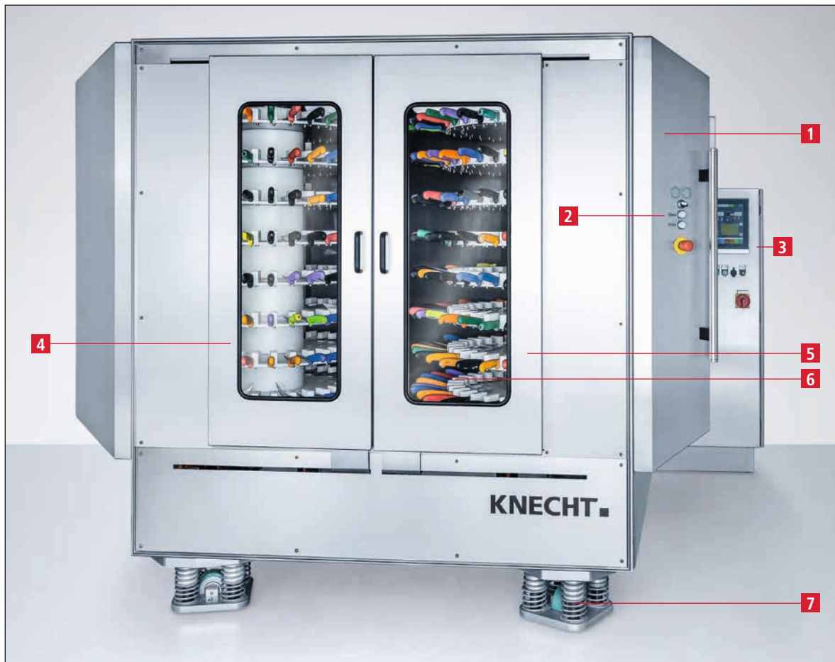
Bild 3-2 Gesamtansicht Schleifmaschine
