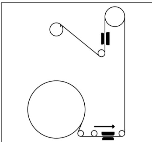
Bild 7-24 Testmedium einsetzen
