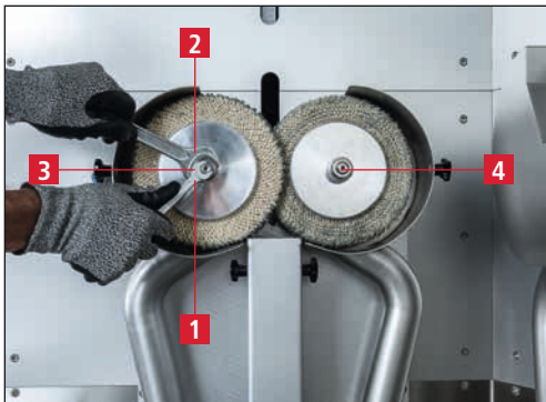
Bild 7-19 Polier-/Entgratringe wechseln
