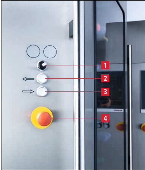
Bild 3-7 Bedienpult Trommelmagazin
