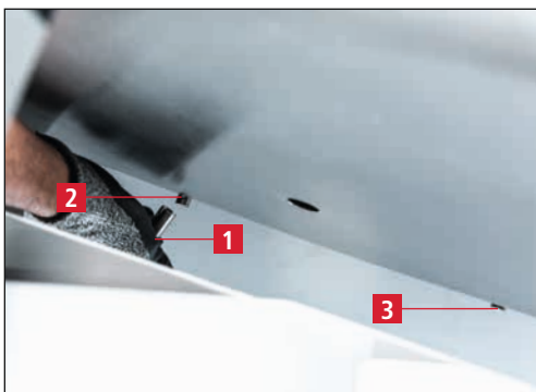
Bild 7-13 Nass-Schleifband ausrichten
