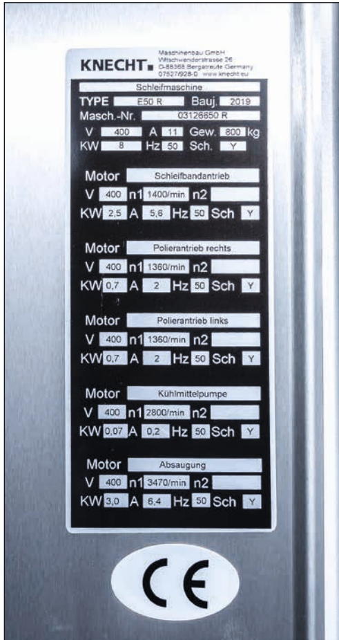
Bild 1-1 Typenschild
