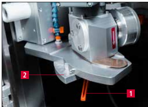
Рис. 7-27 Настройка угла заточки
