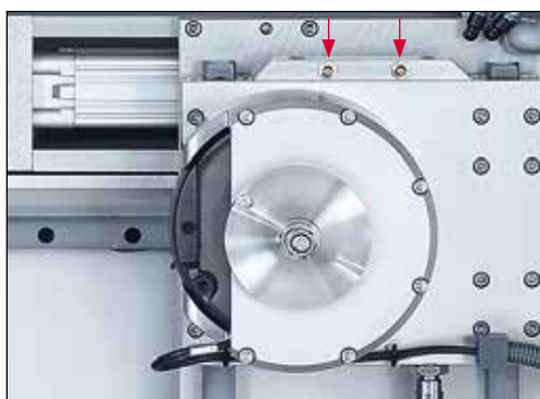
Рис. 9-2 Смазка крестового стола
