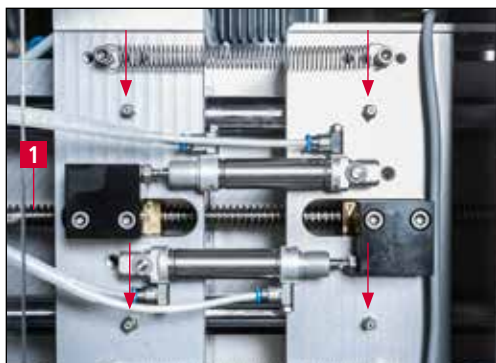
Рис. 9-3 Ось регулировки
