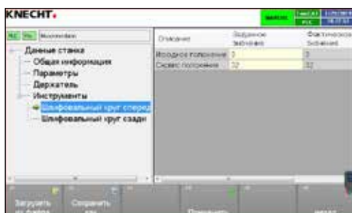
Рис. 8-17 Данные станка «Шлифовальный круг спереди/сзади»
