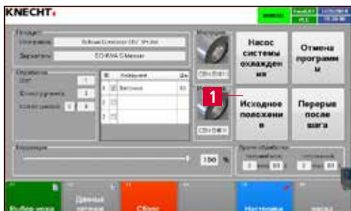
Рис. 7-7 Перемещение кулачкового диска в сменное положение
