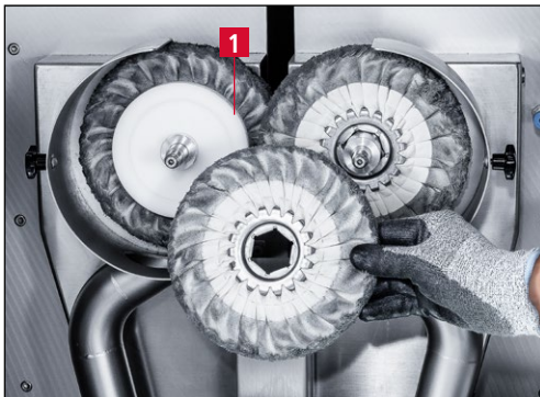
Bild 7-46 Gebrauchten Polierring abnehmen
