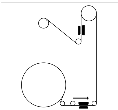
Bild 7-62 Testmedium einsetzen
