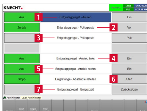
Bild 8-10 Handfunktionen „Entgrataggregat“
