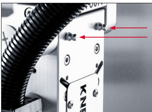
Bild 9-18 Greifer hinten schmieren
