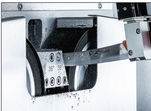
Bild 7-5 Handmesser schleifen
