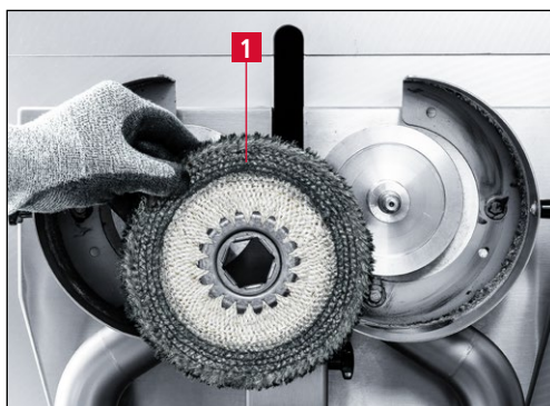
Bild 7-32 Entgratringe wechseln
