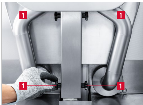
Bild 7-53 Abdeckung öffnen
