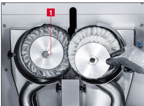
Bild 7-41 Flanschscheibe abnehmen
