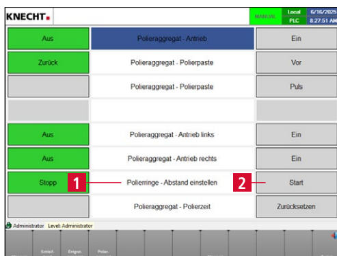
Bild 7-52 Polierringe einstellen
