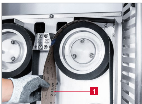
Bild 7-8 Schleifbänder wechseln
