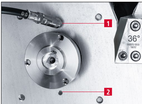
Bild 9-12 Schleifbandmotoren schmieren
