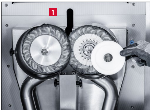
Bild 7-43 Zwischenflansch abnehmen
