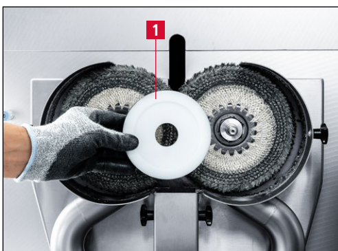
Bild 7-30 Zwischenflansch abnehmen
