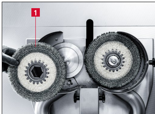
Bild 7-31 Entgratringe wechseln
