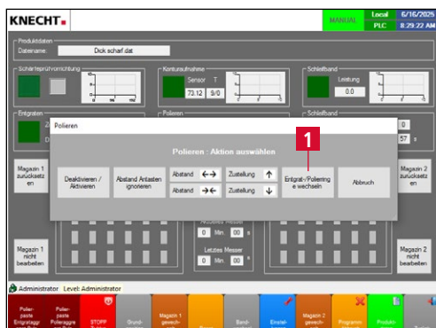
Bild 7-37 Polieren – Polierringe wechseln
