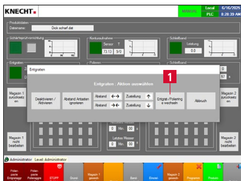
Bild 7-20 Entgraten – Entgratringe wechseln
