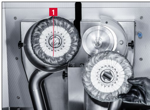
Bild 7-48 Rechten Polierling abnehmen
