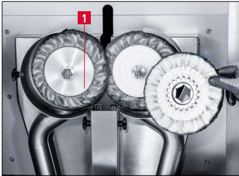
Bild 7-42 Gebrauchten Polierring abnehmen
