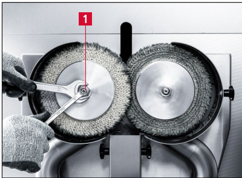
Bild 7-23 Linke Spannmutter abschrauben
