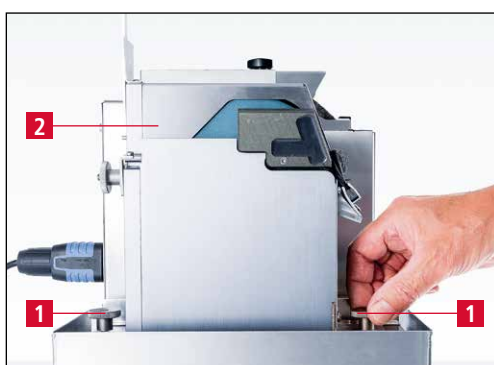
7-6. ábra A késvezető egység levétele
