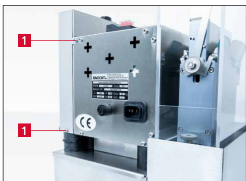
7-10. ábra A polírozótárcsa burkolatának kioldása
