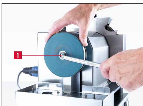
7-7. ábra A csavar meglazítása
