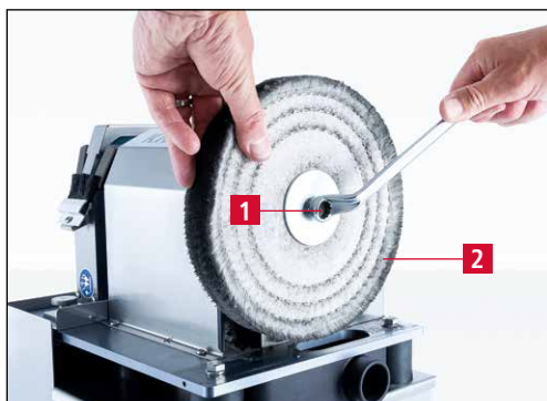
7-13. ábra A polírozótárcsa kioldása
