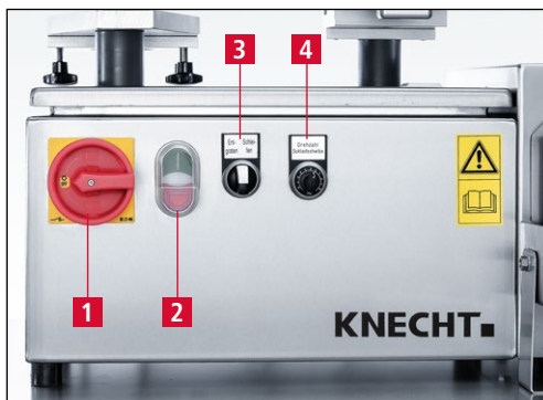
3-4 pav. Valdymo pultas
