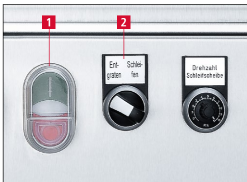
7-86 pav. Diskinių peilių galandimo mašinos įjungimas
