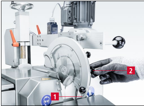
Bild 7-69 Schutzschieber einstellen
