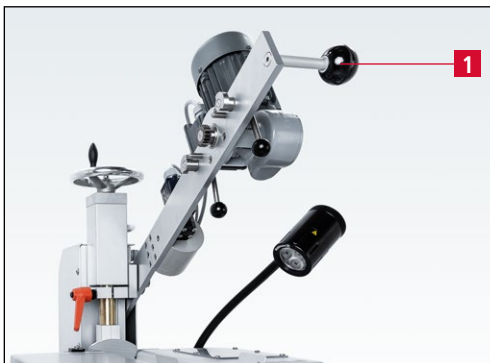
Bild 7-49 Aufnahmearm in Ruheposition
