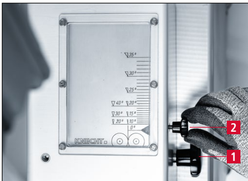
Bild 7-4 Schleifwinkel einstellen
