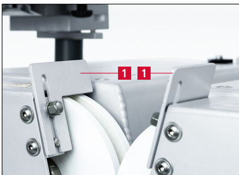
Bild 7-90 Sicherungsschieber montieren
