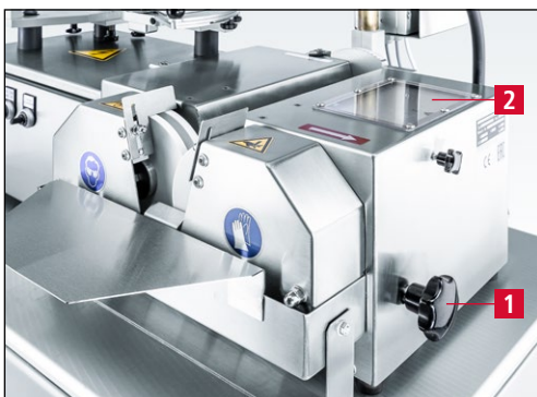
Bild 7-44 Schleifwinkelanzeige
