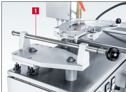
Bild 3-6 Abrichtgerät HV 156
