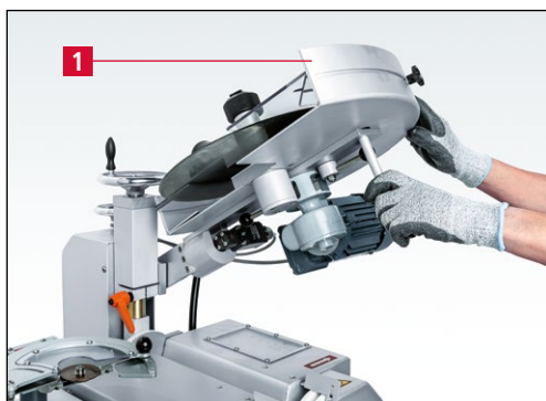
Bild 7-19 Kreismesserschleifeinrichtung nach oben drücken
