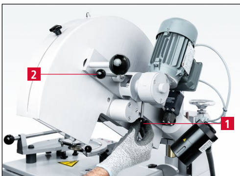
Bild 7-8 Kreismesseraufnahme spannen
