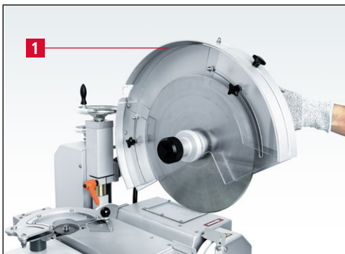
Bild 7-21 Kreismesserschleifeinrichtung in die Schleifposition schwenken
