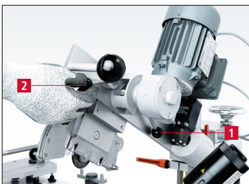
Bild 7-51 Kreismesseraufnahme spannen
