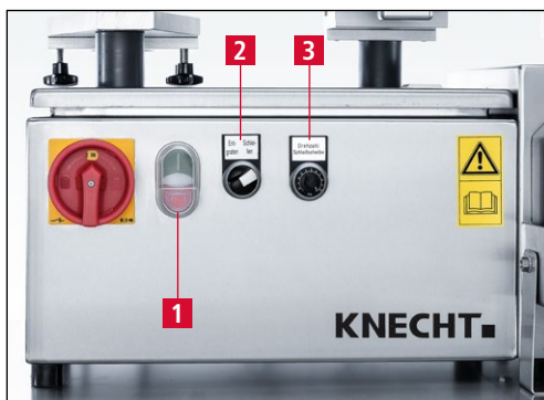
Bild 7-29 Kreismesser-Schärfmaschine einschalten
