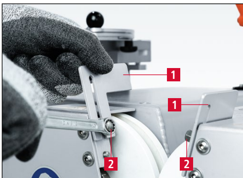
Bild 7-83 Sicherungsschieber entfernen
