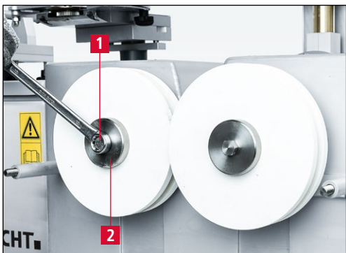
Bild 7-97 Linke Spannschraube lösen
