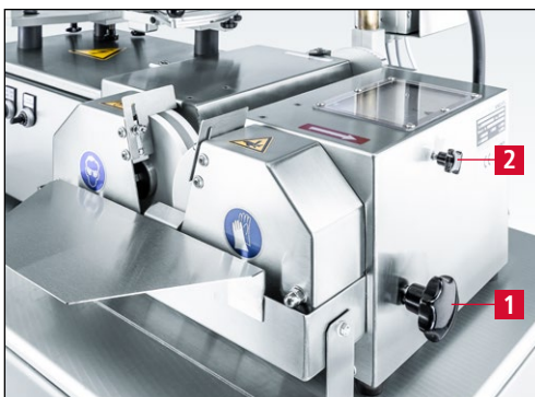
Bild 7-1 Schleifwinkelanzeige
