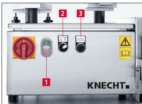
Bild 7-70 Kreismesser-Schärfmaschine einschalten
