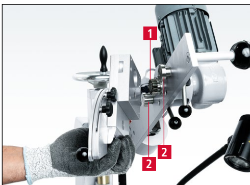
Bild 7-50 Kreismesseraufnahme montieren
