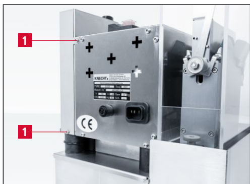
Рис. 7-12 Откручивание крышки полировального круга
