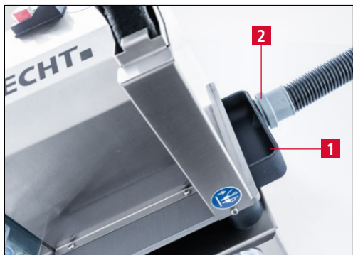
Рис. 7-17 Секция для сбора грязи с отсосным патрубком
