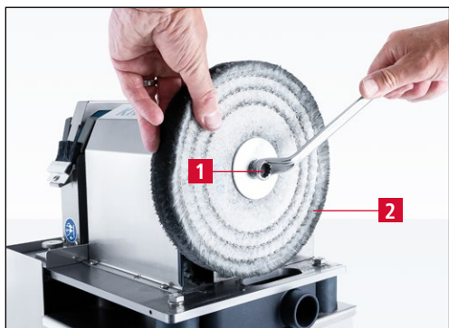
Рис. 7-15 Откручивание полировального круга
