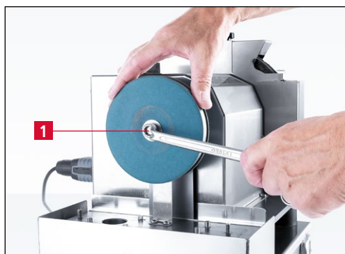
Рис. 7-9 Откручивание болта
