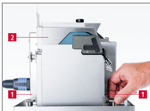
Рис. 7-8 Снятие блока направляющей ножа
