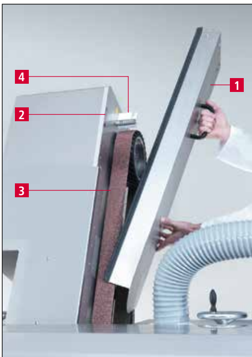
Bild 7-13 Schleifband wechseln
