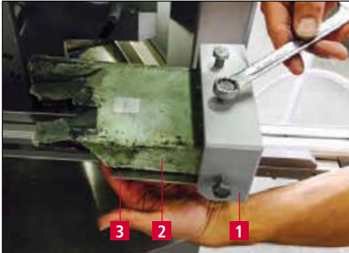
Bild 7-18 Polierpaste wechseln
