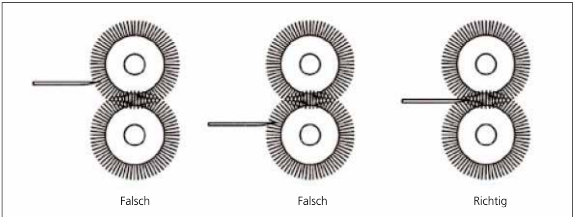
Bild 7-12 Entgrateinheit justieren
