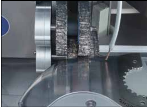
Bild 7-11 Entgrateinheit justieren
