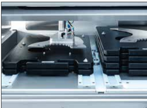
Bild 3-17 Messermagazin mit Messerwechsler
