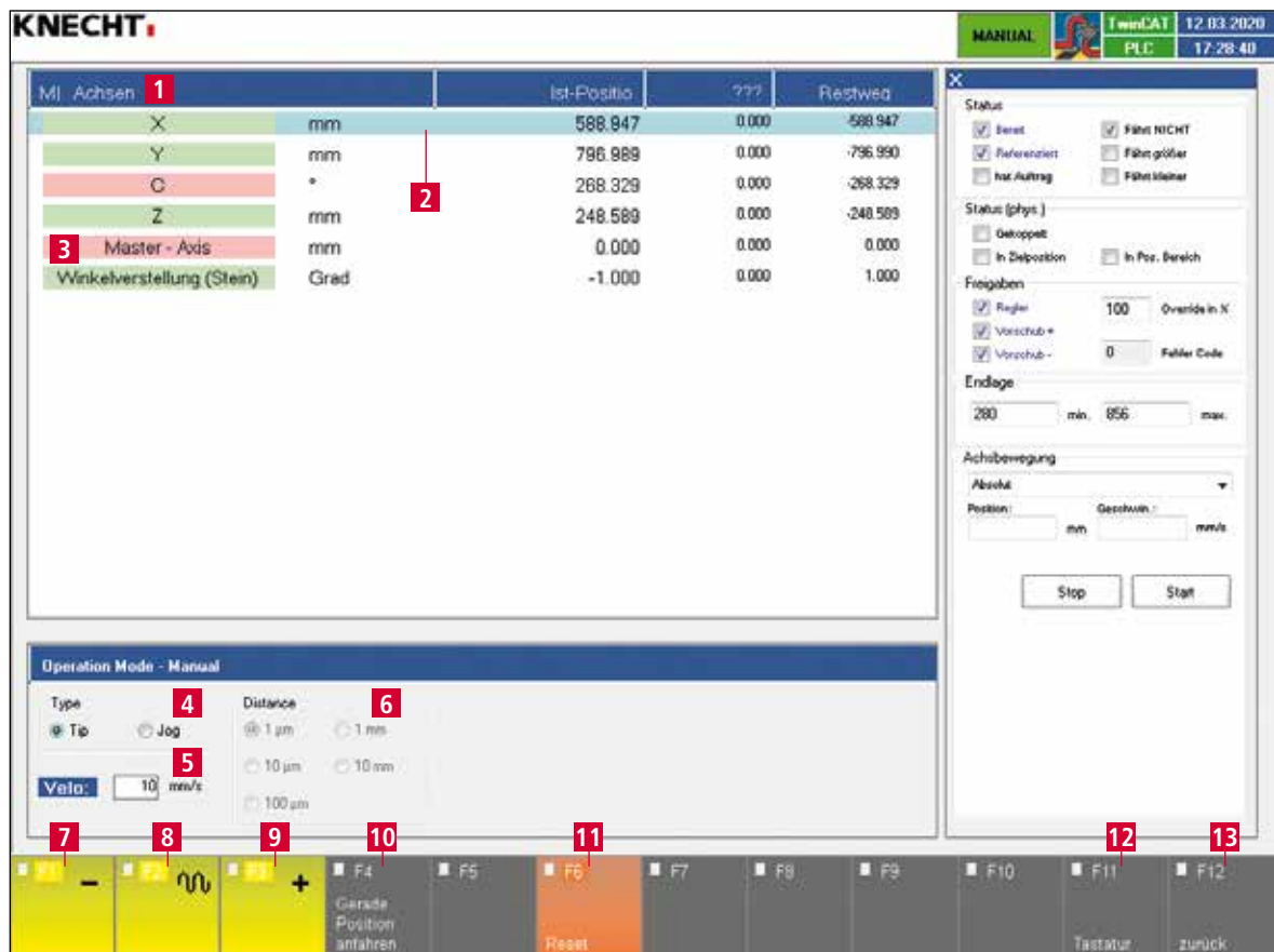
Bild 8-2 Achsen
