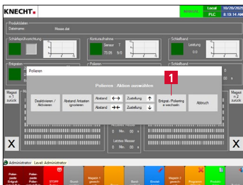
Bild 7-39 Polieren – Polierringe wechseln
