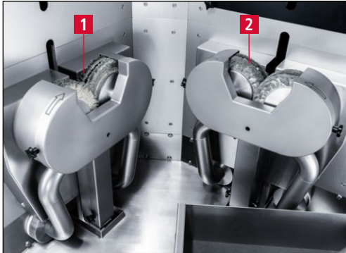
Bild 3-5 Entgrat- und Poliereinheit
