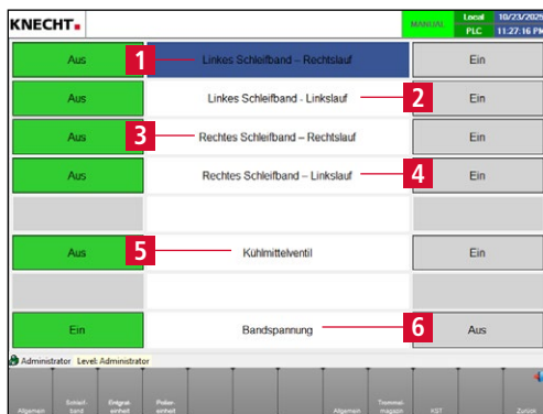
Bild 8-9 Handfunktionen „Schleifband“
