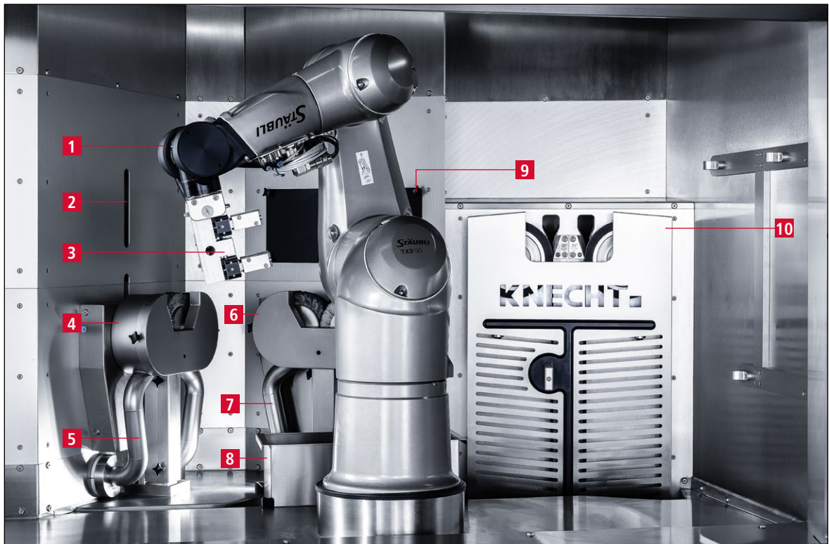
Bild 3-3 Innenraum
