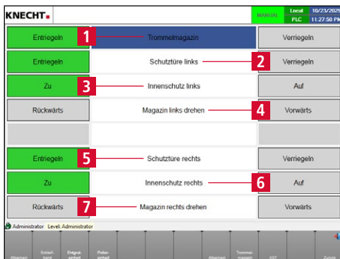
Bild 8-13 Handfunktionen „Trommelmagazin“
