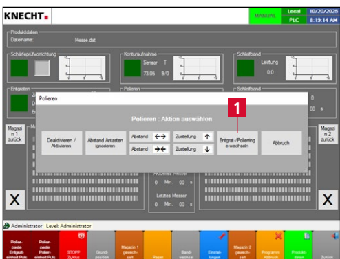
Bild 7-39 Polieren – Polierringe wechseln
