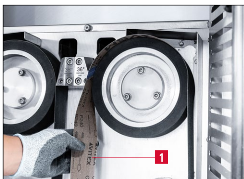
Bild 7-10 Schleifbänder wechseln
