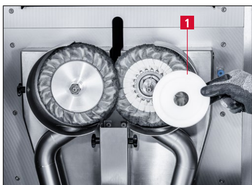
Bild 7-45 Zwischenflansch abnehmen
