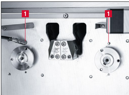
Bild 9-13 Schmiernippel Schleifbandmotoren
