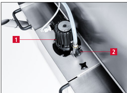
Bild 3-7 Kühlmittelpumpe
