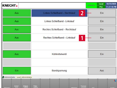
Bild 7-20 Handfunktionen „Schleifband“
