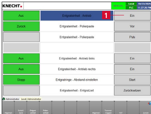
Bild 6-9 Handfunktionen „Entgrateinheit“
