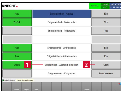
Bild 7-37 Entgratringe einstellen
