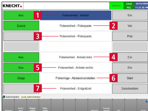
Bild 8-11 Handfunktionen „Poliereinheit“
