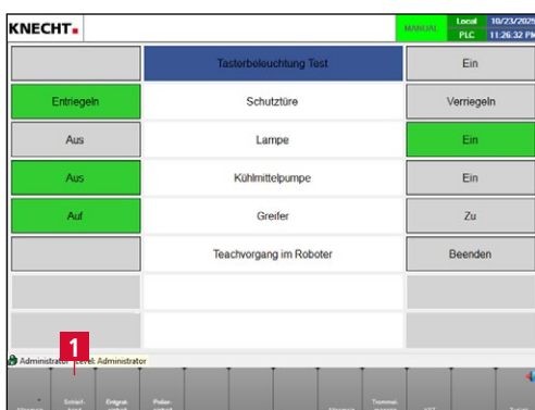
Bild 7-19 Handfunktionen
