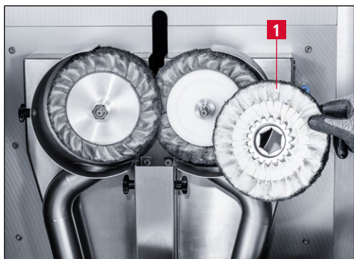
Bild 7-44 Gebrauchten Polierring abnehmen
