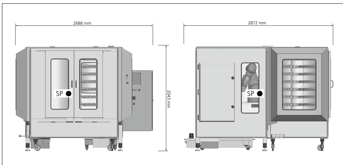
Bild 3-1 Abmessungen in mm und Schwerpunkt (SP) der Maschine
