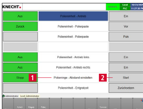
Bild 7-54 Polierringe einstellen
