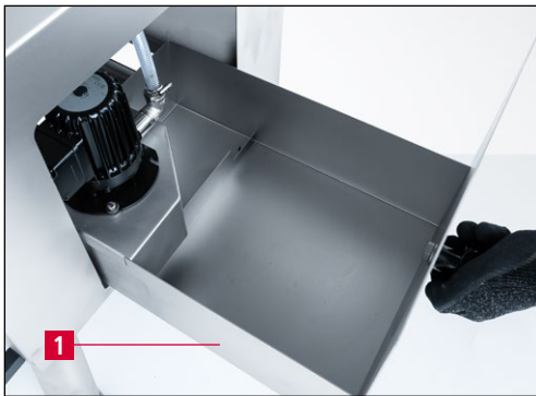
Bild 6-1 Wasserkasten befüllen
